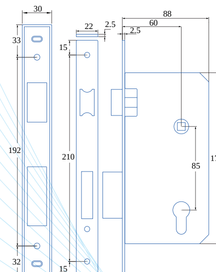
286(60mm) 尺寸圖
