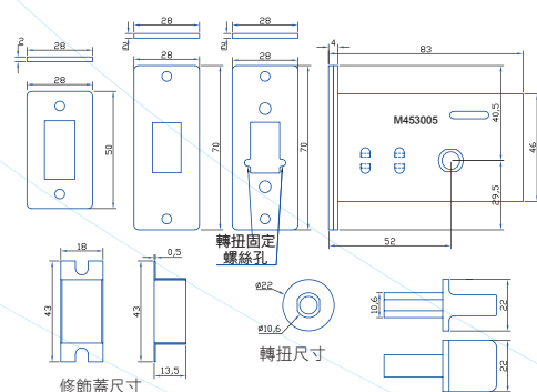
1036鎖匣尺寸圖
