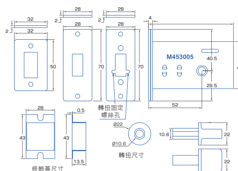
1038鎖匣尺寸圖
