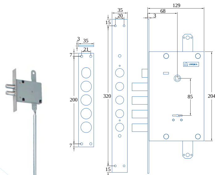
56166 尺寸圖
