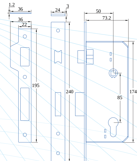
786(50mm) 尺寸圖
