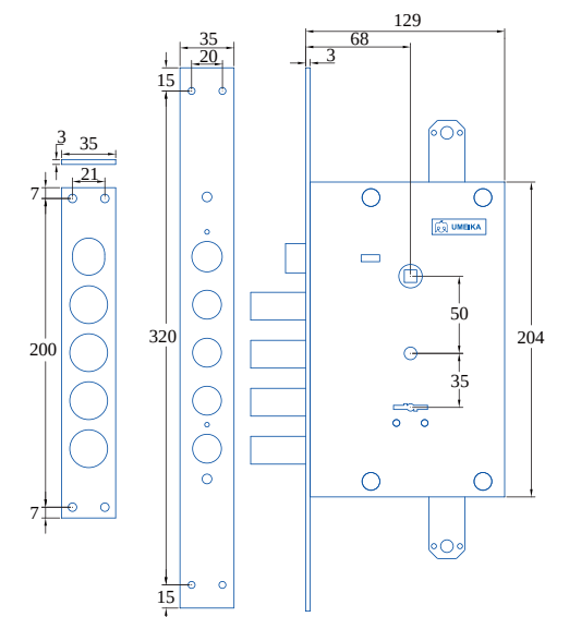
56169 尺寸圖
