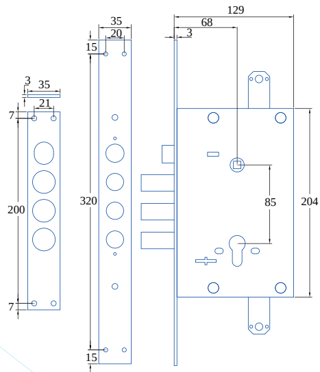
352R 尺寸圖
