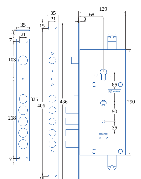
56989 尺寸圖
