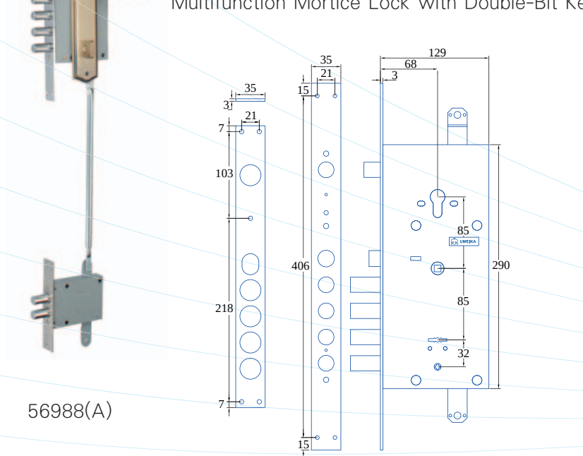
56988 尺寸圖
