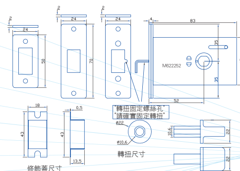
2036鎖匣尺寸圖
