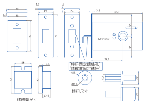
2038鎖匣尺寸圖
