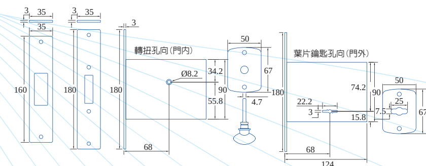
SL-04 尺寸圖
