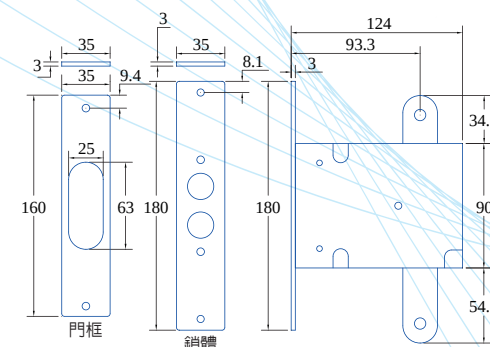
SL-01 尺寸圖
