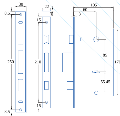
186(雙插式) 尺寸圖
