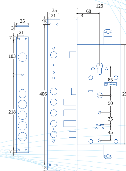
56988 尺寸圖
